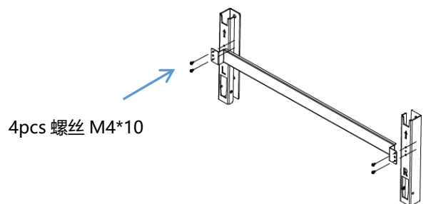
挂板组装示意图
