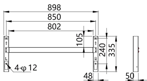
挂板尺寸
